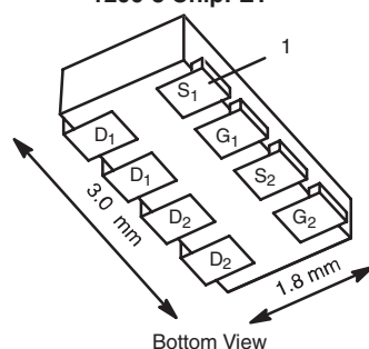
1206-8 ChipFET®
